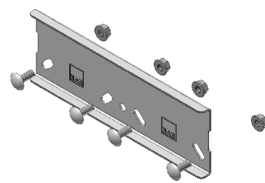
060 UKS Ek Elemanı
